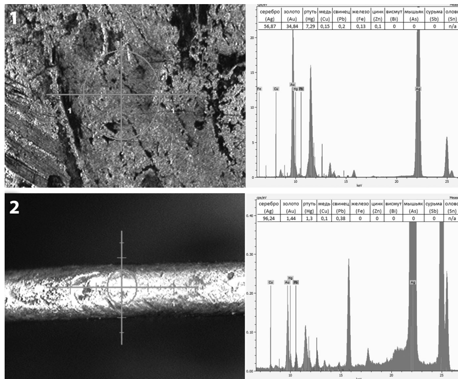
Рис. 10. Результаты РФА состава металла дирхема неизвестного происхождения: 1 – слой позолоты на аверсе, 2 – гурт со стертой позолотой
