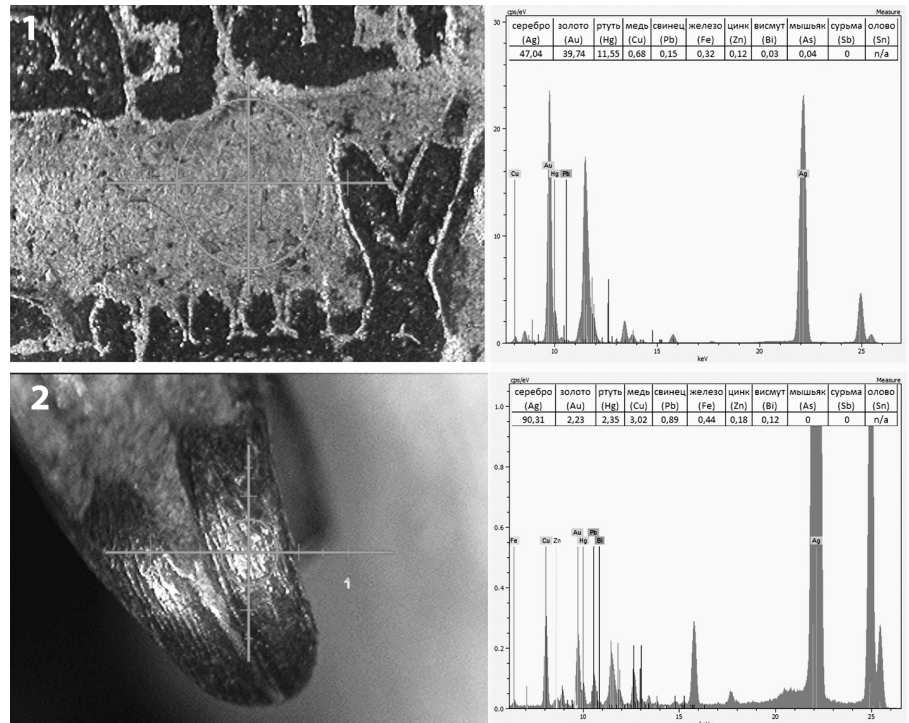
Рис. 3. Результаты РФА состава металла дирхема-подвески из Гнездова: 1 – слой позолоты на аверсе, 2 – ушко с остатками позолоты
