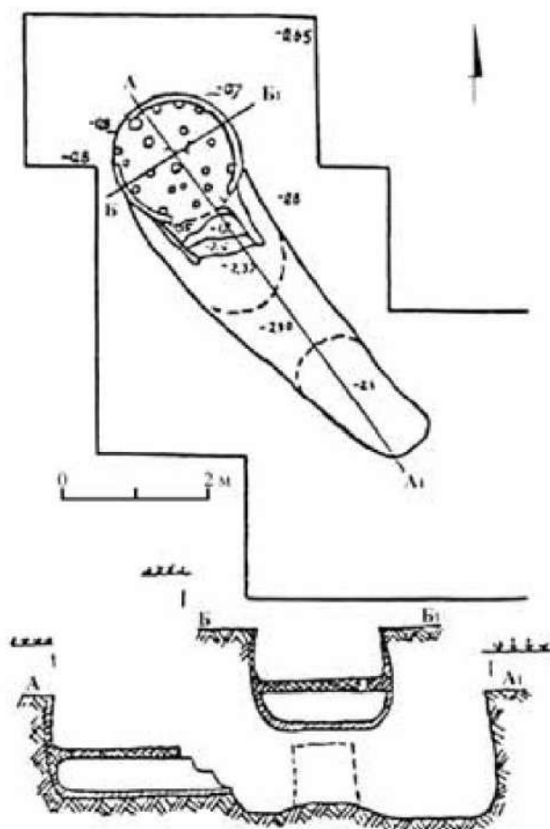
Рис. 13. Гончарный горн с селища Каменное (по: Сухобоков, 2016. С. 68)
