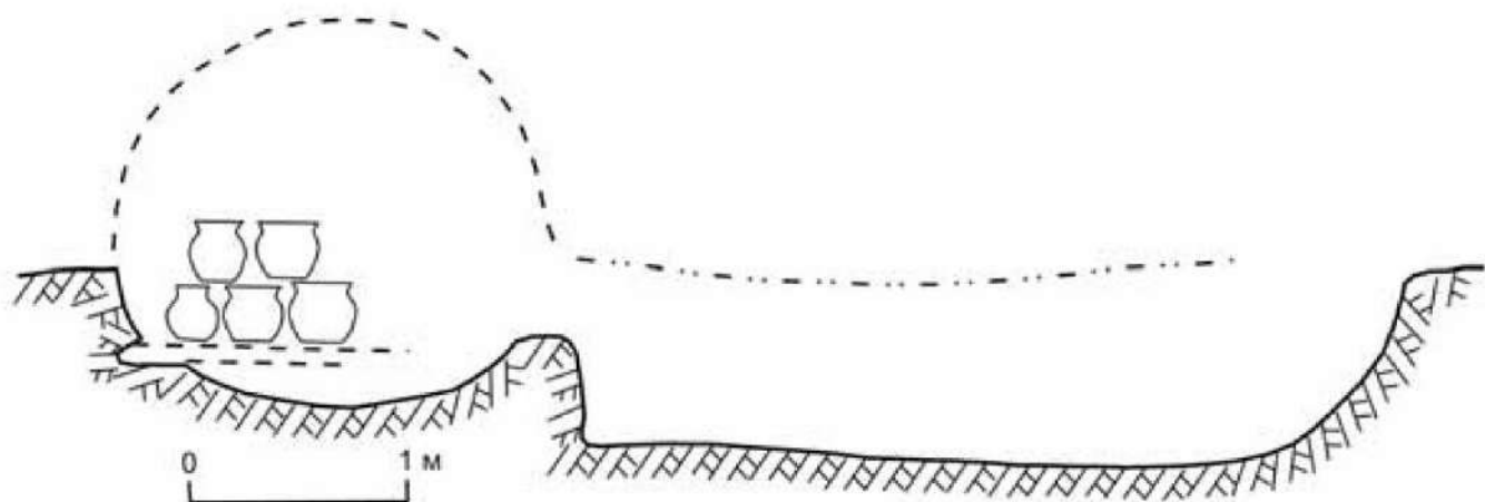
Рис. 10. Реконструкция продольного разреза гончарного горна на Гнёздовском селище (по линии запад–восток)
