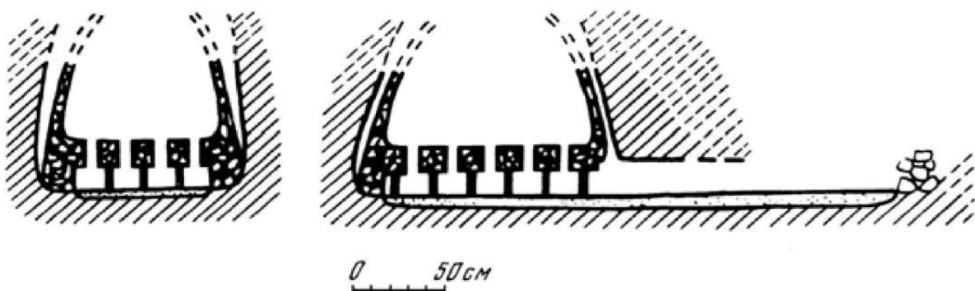
Рис. 14. Гончарный горн с поселения Асардаре-Плиска (по: Бобринский, 1991. С. 105)
