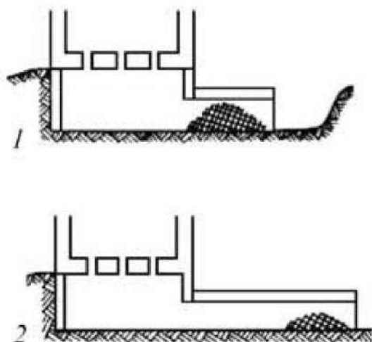
Рис. 11. Топка периферического действия (1) и топочный канал с функцией воздушно-тягового устройства (2) по классификации А.А. Бобринского (типы СТП-2 и СТП-3) (по: Бобринский, 1991. С. 116)
