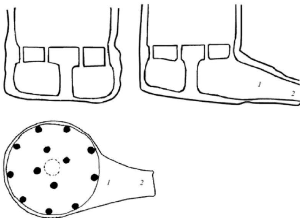
Рис. 17. Типовая схема горна из балки Канцерка. На схеме обозначены камера для сжигания топлива (1), загрузочное устройство для топлива (2) (по: Володарець-Урбанович, 2011. С. 33)
