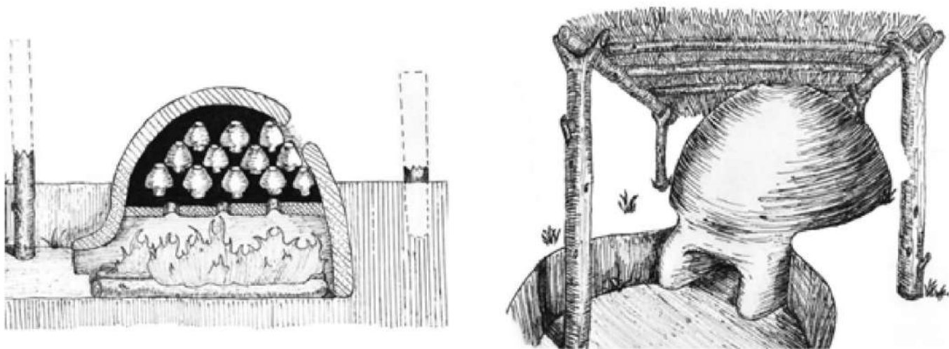
Рис. 15. Графическая реконструкция гончарного горна с посада Вышгорода (по: Готун и др., 2013. С. 149)
