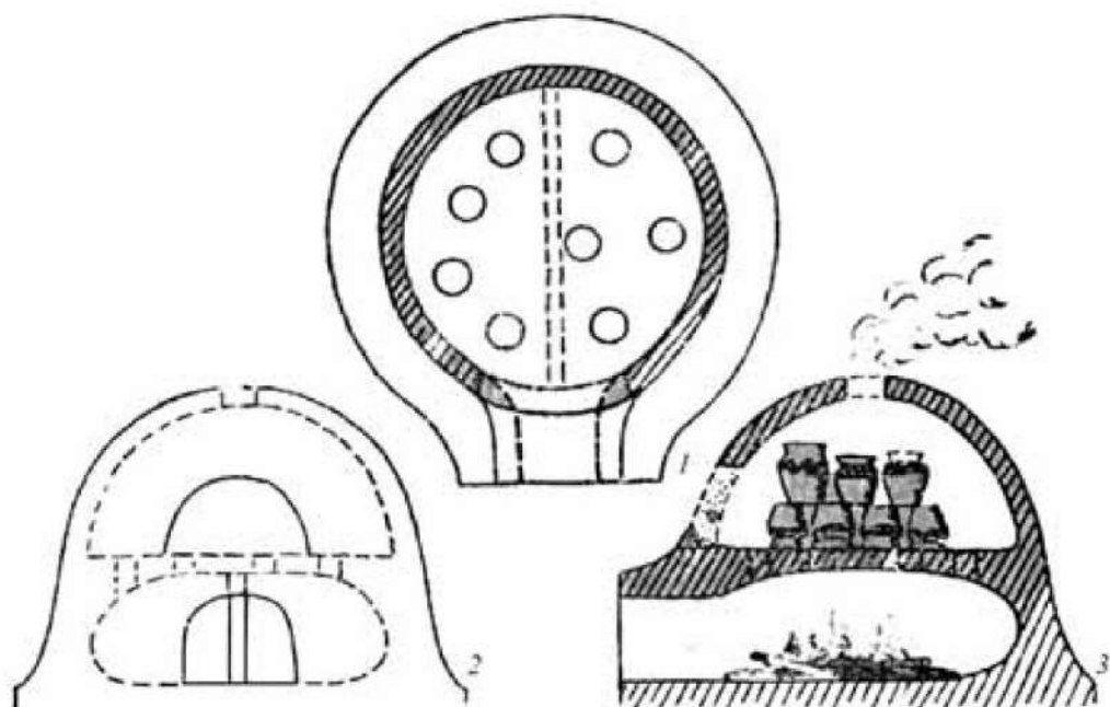
Рис. 16. План (1), разрез (2) и графическая реконструкция (3) гончарного горна с Донецкого городища (по: Шрамко, 1962. С. 341)
