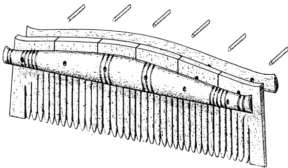
Рис. 2. Схема сборки рогового одностороннего составного гребня (по: Ambrosiani, 1984).
